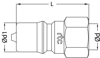
Plug / Nippel
