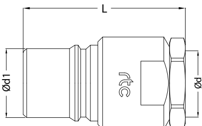
Plug / Nippel
