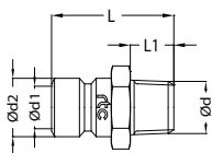
Plugs / Nippel
