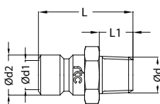
Plugs / Nippel
