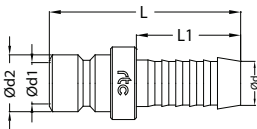
Plugs / Nippel
