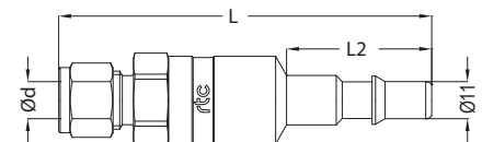
Stainless steel tube connection plug with valve Verschlussnippel mit Edelstahlrohranschluss
