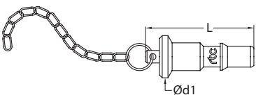
Sockets dust cup Kupplungstaubschutzkappe
