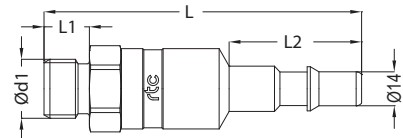
Male thread plug with valve Verschlussnippel mit Aussengewinde
