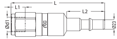
Female thread plug with valve Verschlussnippel mit Innengewinde
