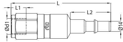
Female thread plug with valve Verschlussnippel mit Innengewinde
