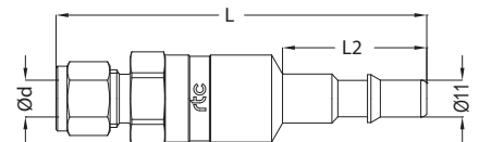
Copper tube connection plug with valve Verschlussnippel mit Kupferrohranschluss
