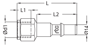
Female thread plug Nippel mit Innengewinde
