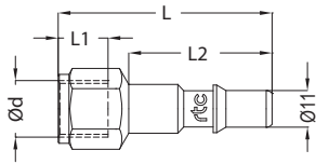
Female thread plug Nippel mit Innengewinde
