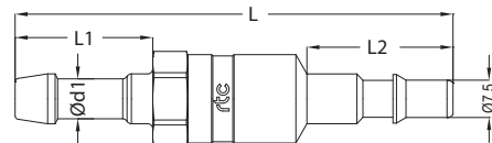
Standard hose tail plug with valve Verschlussnippel mit Schlauchanschluss
