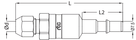
Plastic hose connection plug with valve Verschlussnippel mit Anschluss für Kunststoffschlauch
