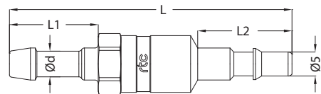
Standard hose tail plug with valve Verschlussnippel mit Schlauchanschluss
