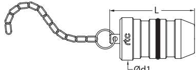
Plug dust cup Stecknippelsschutz
