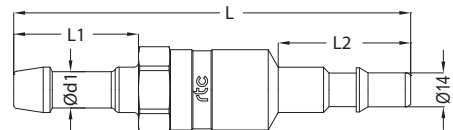
Standard hose tail plug with valve Verschlussnippel mit Standard - Schlauchtülle
