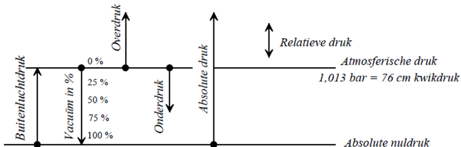
Figuur 3.24: Verschillende mogelijke referenties bij drukmetingen.
